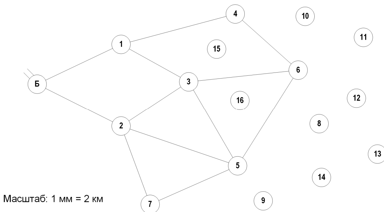
Рисунок – 1 Карта-схема размещения подстанций
