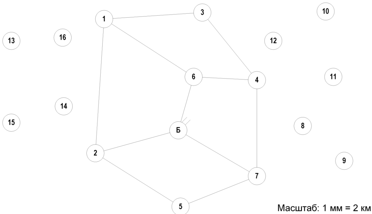
Рисунок – 1 Карта-схема размещения подстанций
